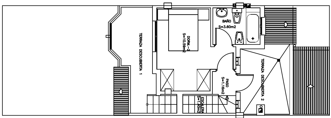
PLANTA PRIMERA
