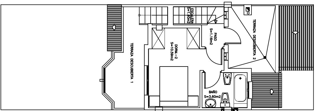
PLANTA PRIMERA
