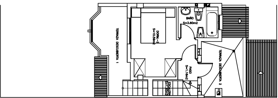
PLANTA PRIMERA
