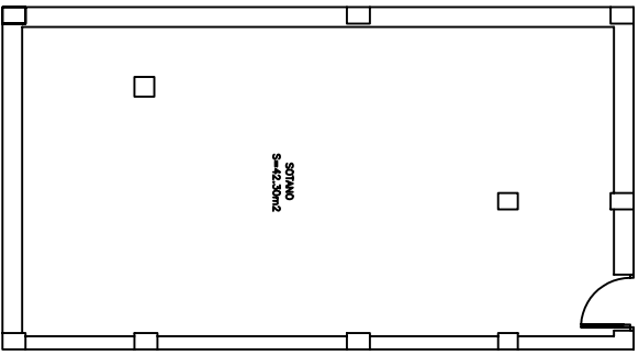
PLANTA SOTANO
