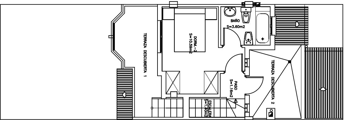
PLANTA PRIMERA
