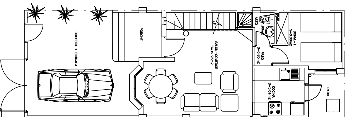
PLANTA BAJA
