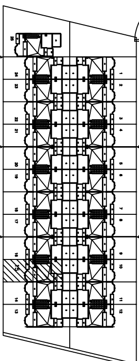
PLANTA PRIMERA
