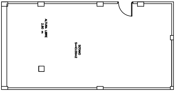
PLANTA SOTANO
