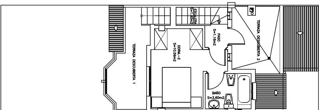
PLANTA PRIMERA
