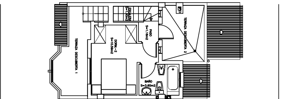
PLANTA PRIMERA
