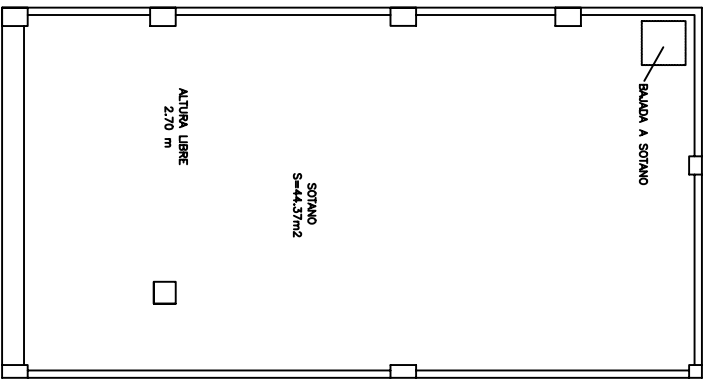
PLANTA SOTANO
