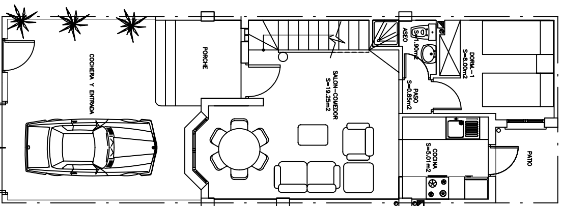
PLANTA BAJA
