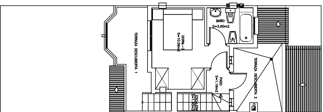
PLANTA PRIMERA
