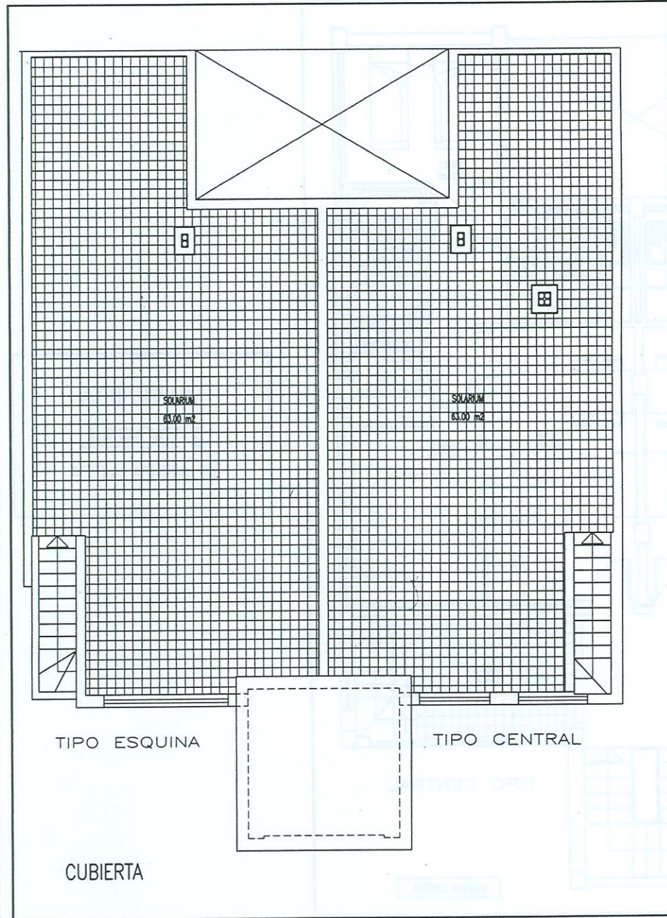
Cubierta/Roof (2 Dormitorios/2Bedrooms)
